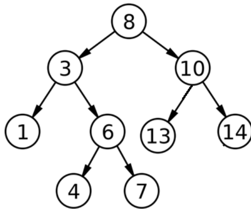
Рис.1. Бинарное дерево поиска
